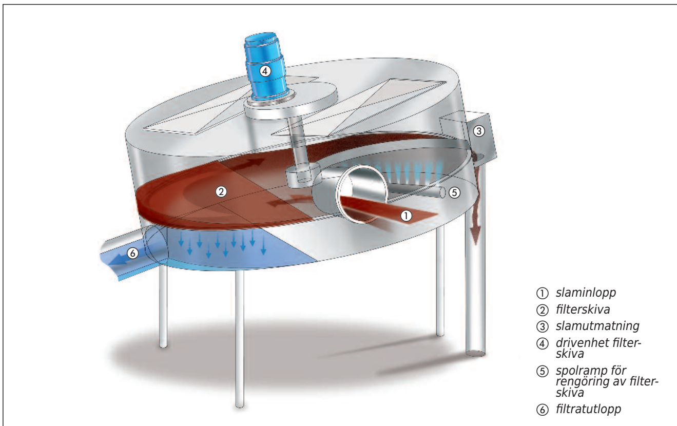
Schematisk bild över ROTAMAT® skivfilter RoS 2S
