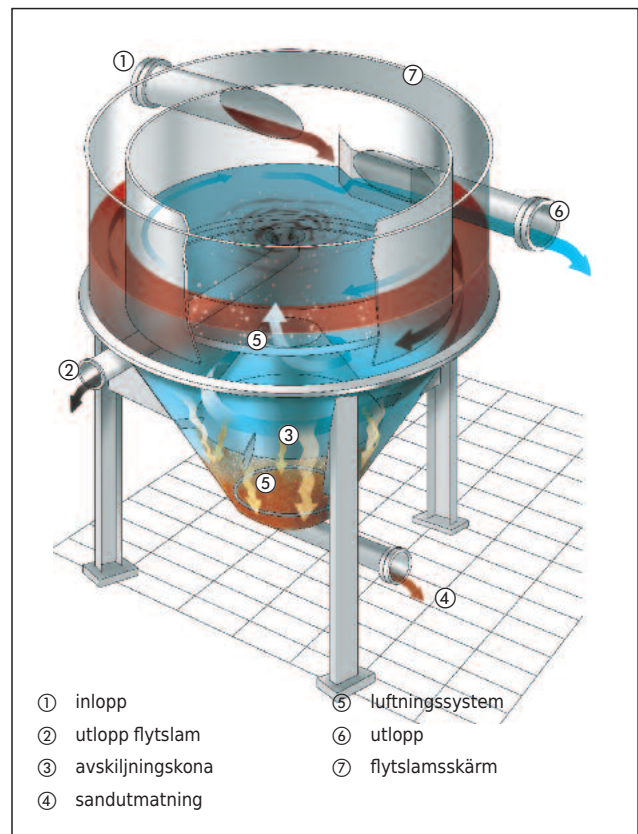
Flödesdiagram HUBER Rundsandfång HRSF
